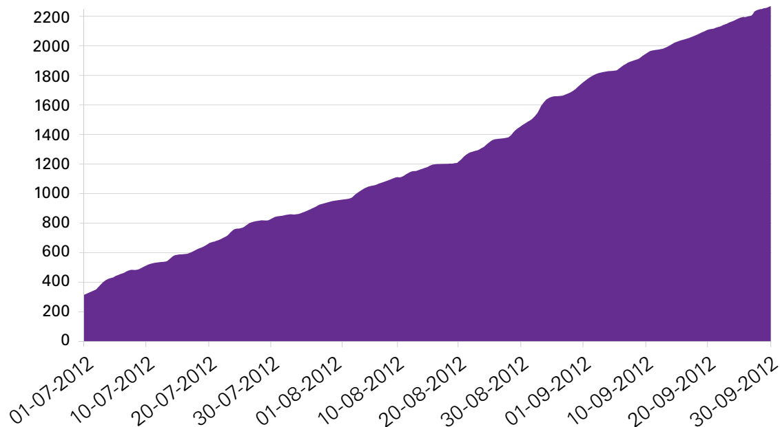
Liczba nazw domeny .pl zabezpieczonych protokołem DNSSEC w trzecim kwartale 2012
